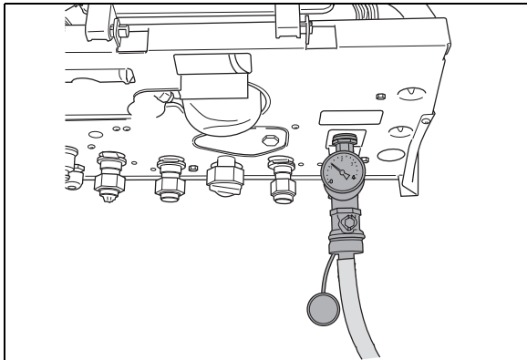
Рис. 7 Выпуск воды из отопительной установки
